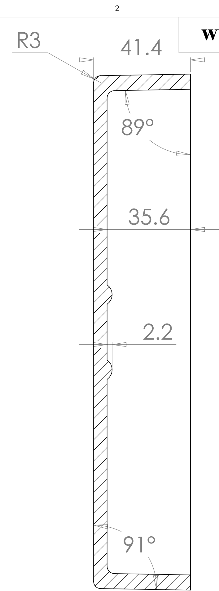
SECTION A-A SCALE 1:1
